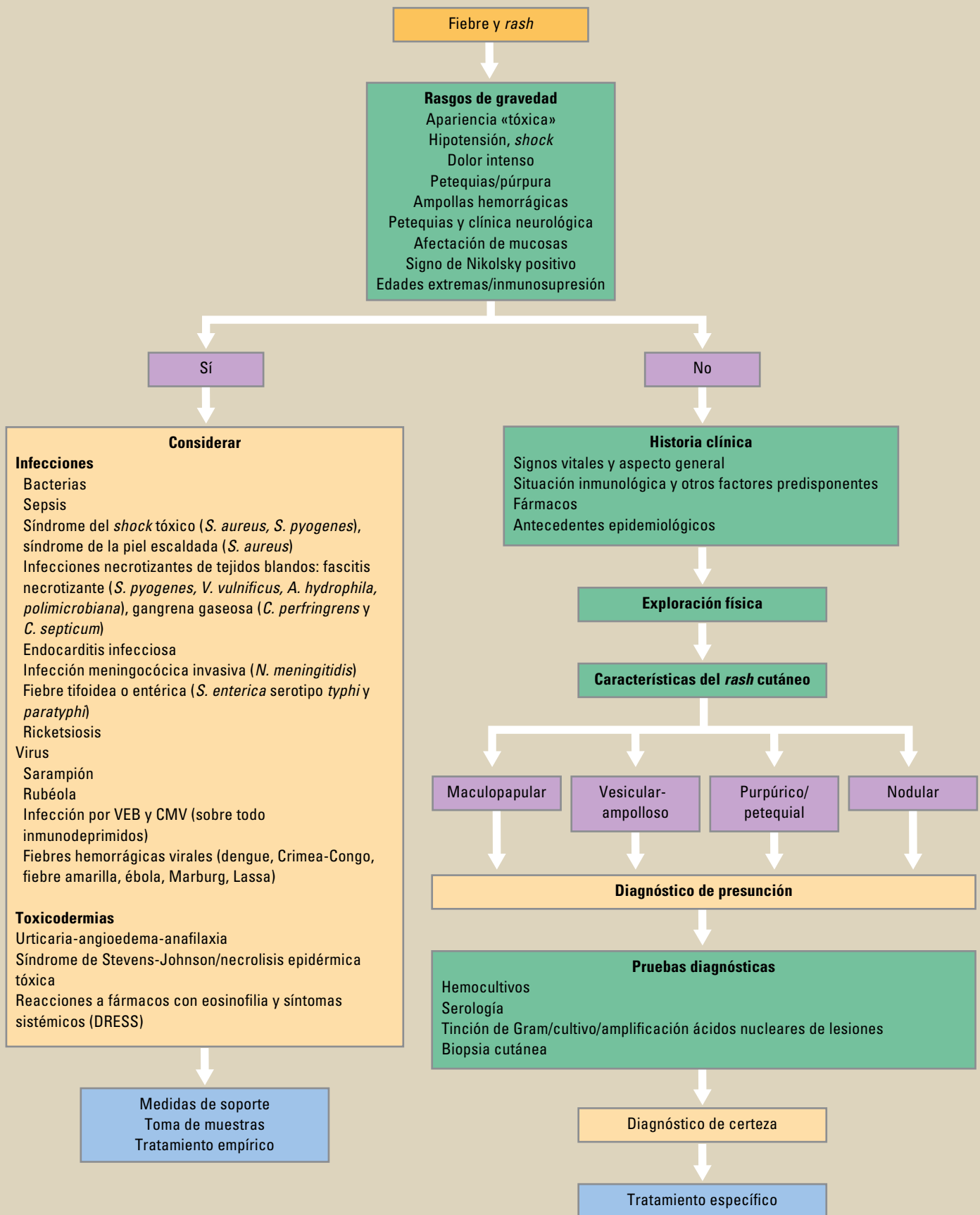
Fig. 1. Algoritmo diagnóstico ante un paciente con fiebre y rash cutáneo.
