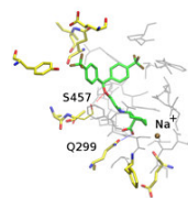
mGAT2 preference
