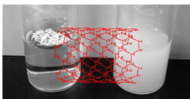
BNNTs BNNT-DSPE-PEG2000
