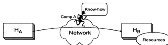
Fig. 2. MA paradigm.
