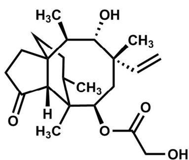
pleuromutilin ( 31 )
