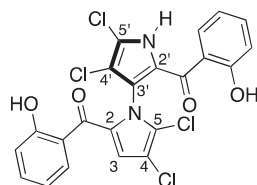
(-)-marinopyrrole A, (-)-1
