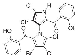
(-)-marinopyrrole B, (-)-2
