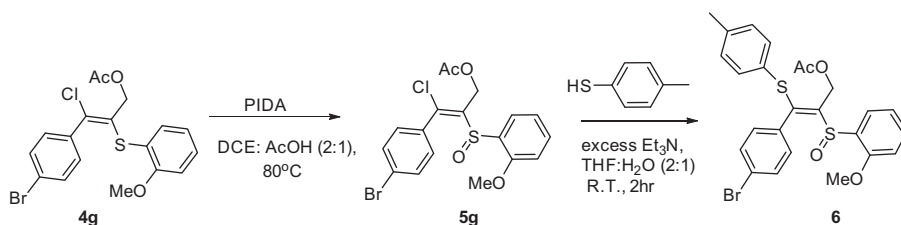
Scheme 2. Synthesis of ( E )-3-(4-bromophenyl)-2-((2-methoxyphenyl)sulfinyl)-3-( p -tolylthio)allyl acetate 6 .
