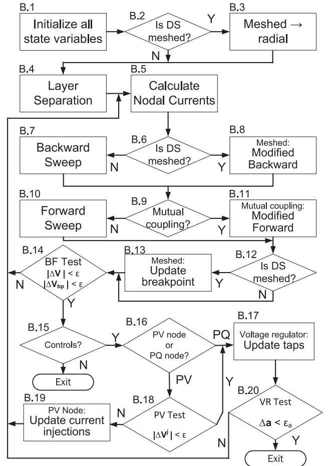
Fig. 2. BFS algorithm.
